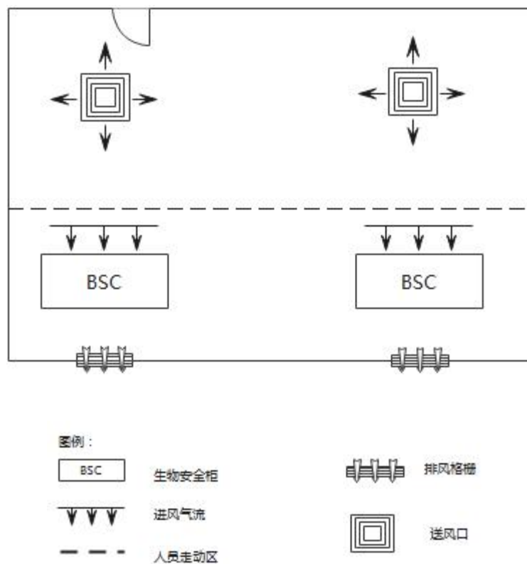
图 A.1 A2 型生物安全柜在有气流控制的生物安全二级实验室安装位置示例
